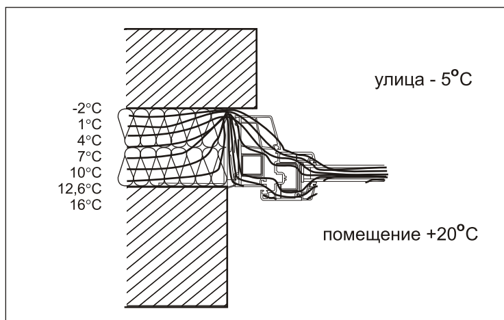
Рис. 37: Двойная бетонная стена с внутренней изоляцией и вентиляцией, пластиковое окно с коробкой в области изоляции
