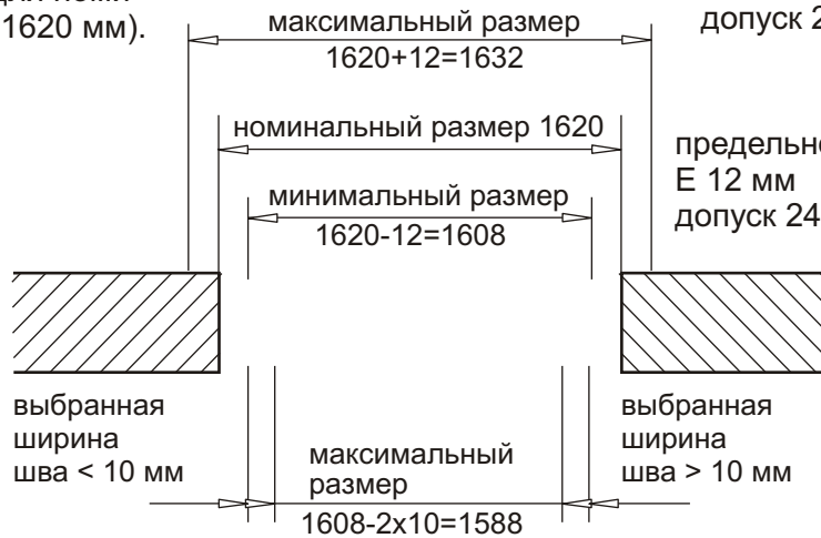
Рис. 4: Пригонка оконных рам
