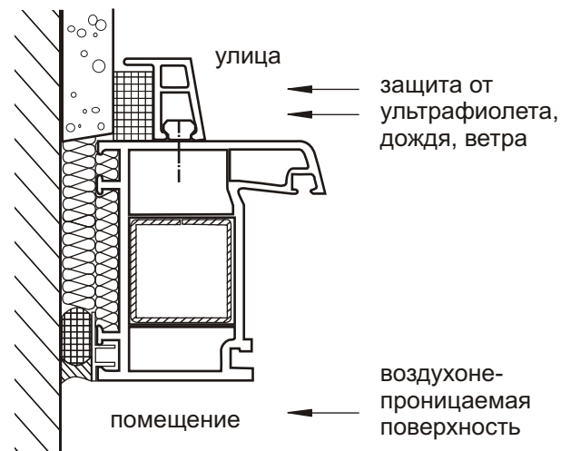
Рис. 27: Двухступенчатое исполнение шва
