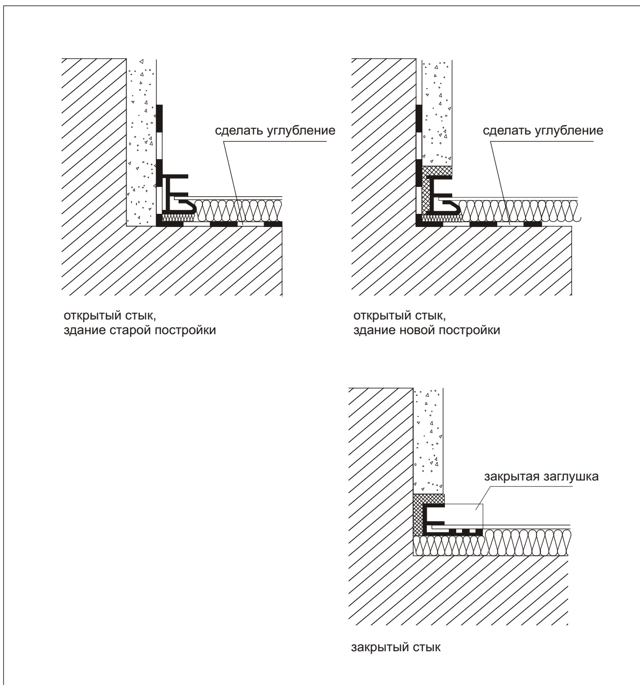
Рис. 33: Герметизация боковых частей сливов и подоконников
