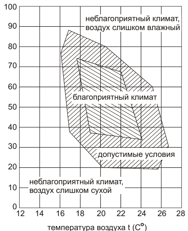
Рис. 34: Диаграмма Лейсдена-Фреймарка
