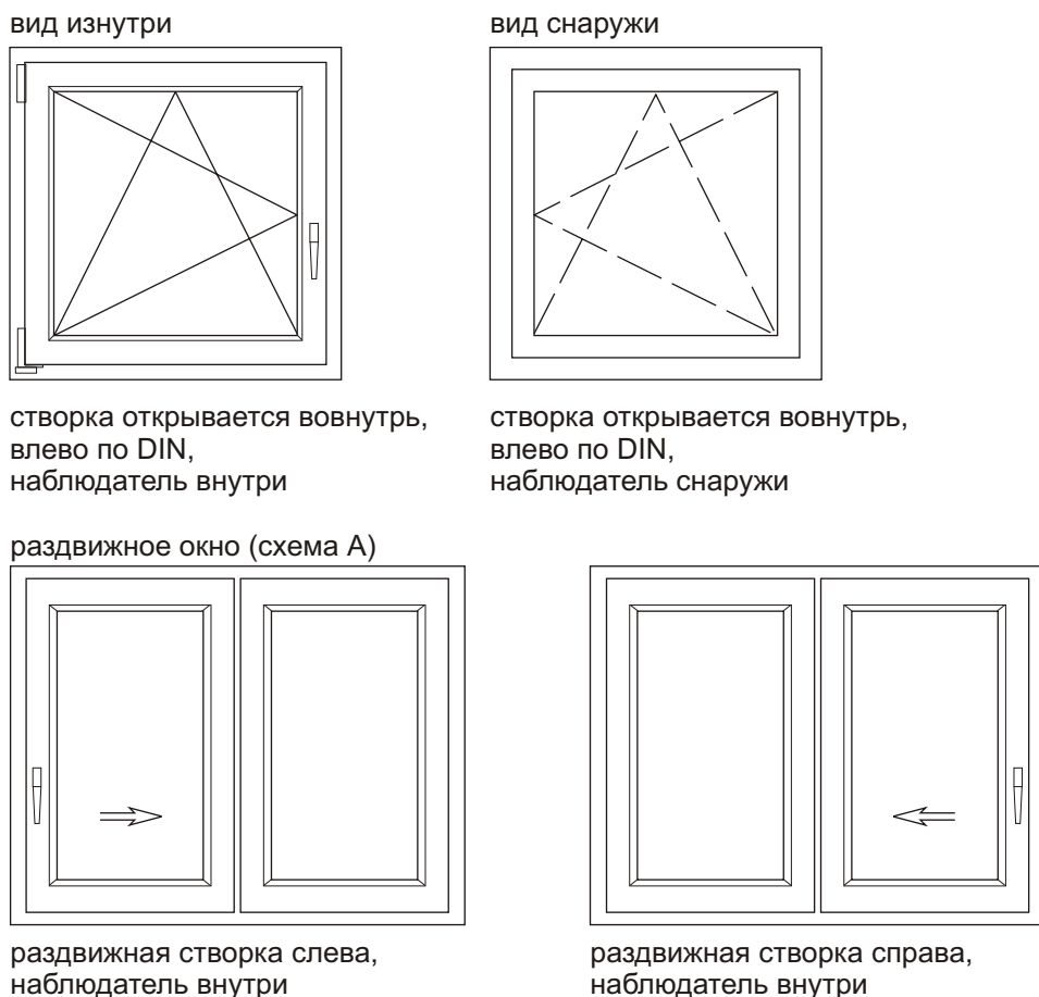
Рис. 8: Виды окон
